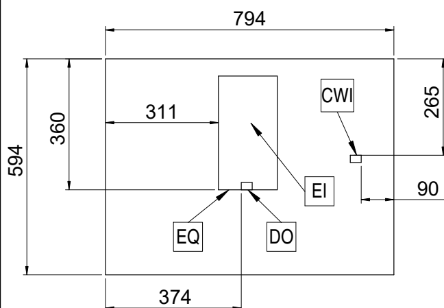
Dessus
